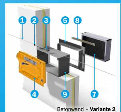
Betonwand - Variante 2
