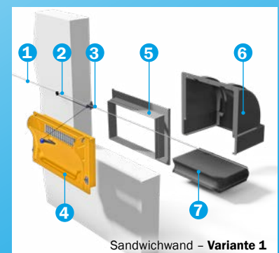
Sandwichwand - Variante 1
